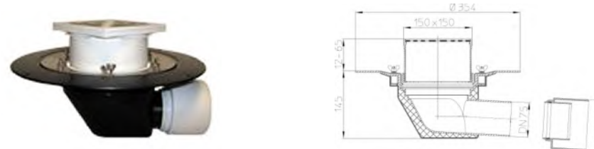
Рис. 1. Кровельная воронка HL64B.
